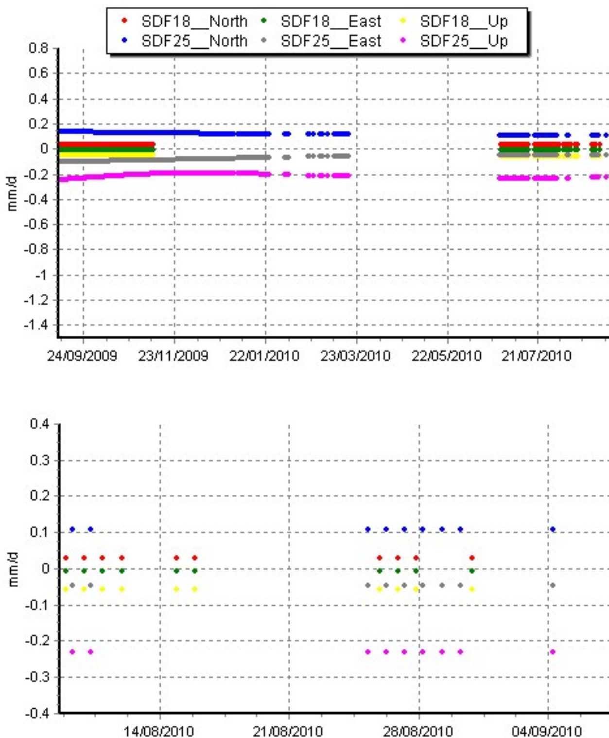
Fig. 3.2 Variazione delle Velocità di Deformazione verticale e orizzontale (nelle due componenti Nord e Est) di due capisaldi del sistema THEODOROS (SDF18 e SDF25). Le velocità, medie giornaliere, sono misurate in mm/giorno. I periodi considerati nei grafici sono di un anno (in alto) ed un mese (in basso).
