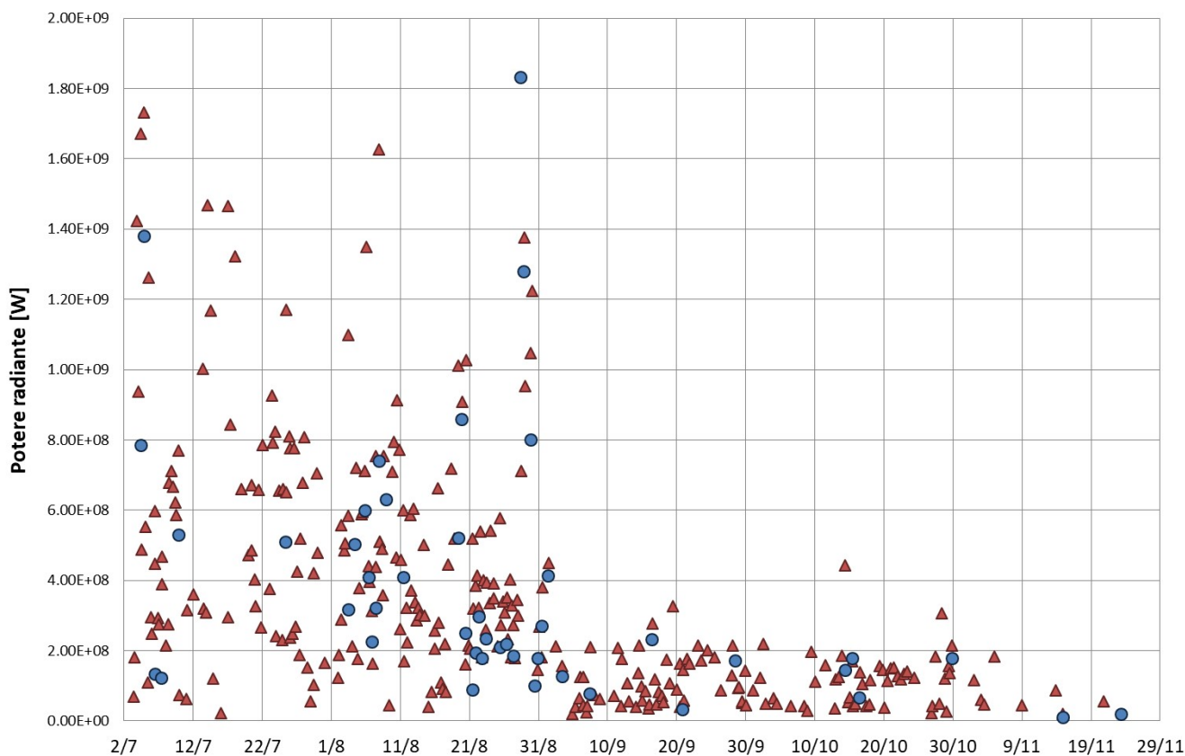
Fig. 7.1 - Flusso radiante calcolato da dati MODIS (triangolo rosso) e Sentinel-3 SLSTR (cerchio blu) dal 3 luglio al 23 novembre.
