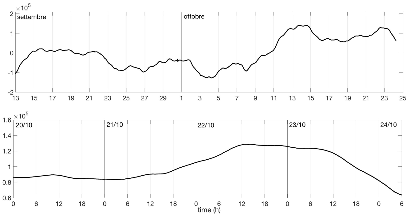
Fig. 4.3 - Grafico relativo al dato dilatometrico registrato alla stazione SVO: in alto viene mostrato lo strain registrato dal 13/09/2019, in basso quello nell'ultima settimana.
