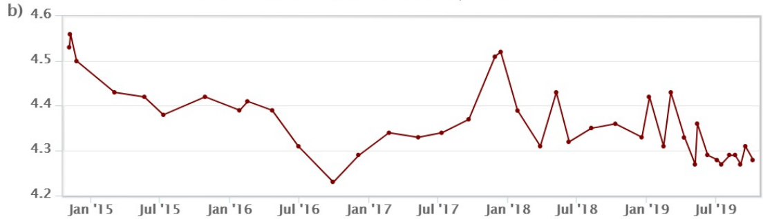
Fig. 6.3 - Andamento temporale medio del rapporto isotopico dell'elio disciolto nella falda termale: a) ultimo anno; b) ultimo quadriennio.
