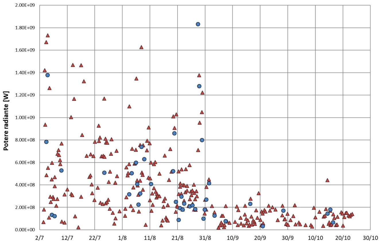
Fig. 7.1 - Flusso radiante calcolato da dati MODIS (triangolo rosso) e Sentinel-3 SLSTR (cerchio blu) dal 3 luglio al 23 ottobre.
