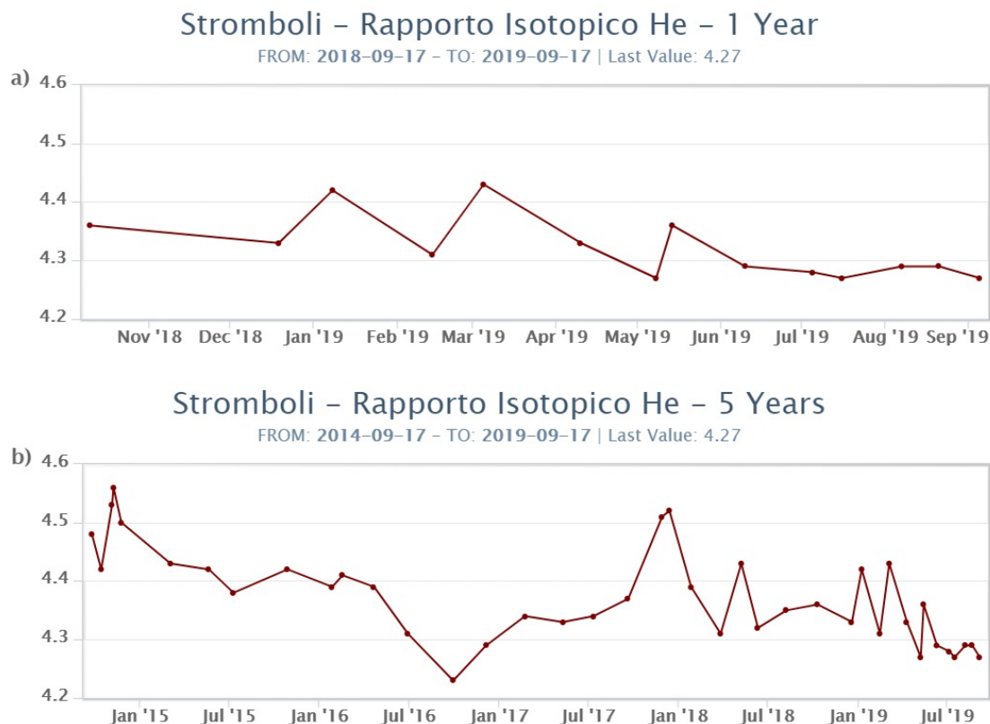
Fig. 6.2 - Andamento temporale medio del rapporto isotopico dell'elio disciolto nella falda termale: a) ultimo anno; b) ultimo quadriennio.
