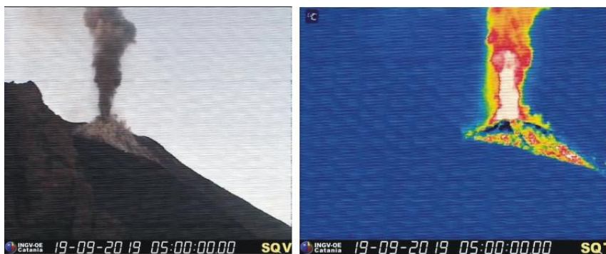
Fig. 3.1 - Immagini visibile (a sinistra) e termica (a destra) dell'attività stromboliana dalle bocche presenti nell'area craterica N; il materiale grossolano ricade lungo i fianchi del cono prospiciente la Sciara del Fuoco. Immagini delle telecamere di quota 400 m del 19 settembre 2019.
