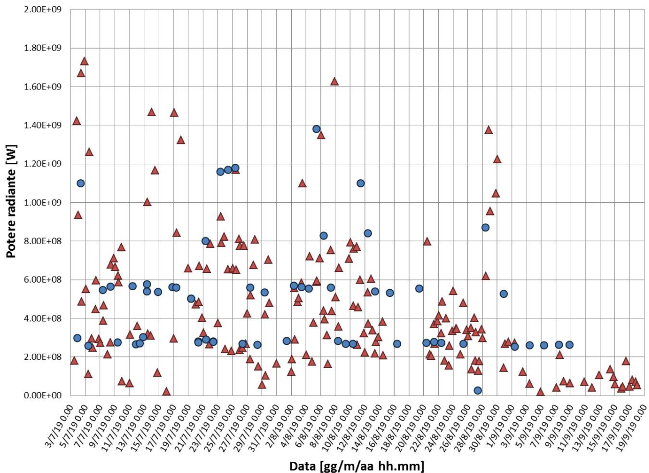
Fig. 7.1 - Flusso radiante calcolato da dati MODIS (triangolo rosso) e Sentinel-3 SLSTR (cerchio blu) dal 3 luglio al 18 settembre.
