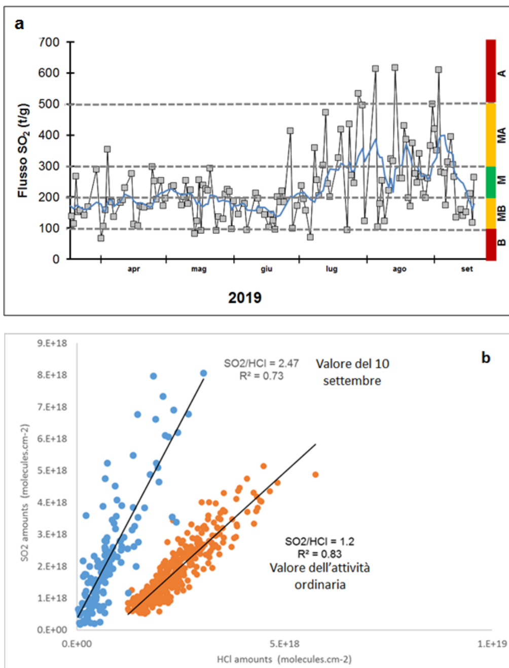
Fig. 6.1 - Andamento temporale del flusso di SO 2 nel corso dell'ultimo semestre (a) Livelli di degassamento: B=Basso, MB=Medio-Basso, M=Medio, MA=Medio-Alto, A=Alto. in (b) rapporto SO 2 /HCl, in blu: valore misurato il 10 settembre in arancione il valore tipico misurato durante l'ordinaria esplosiva dello Stromboli.
