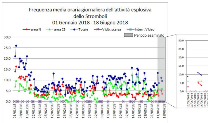
Fig. 3.2 - Nel grafico è visualizzata la frequenza oraria media giornaliera degli eventi esplosivi ripresi
