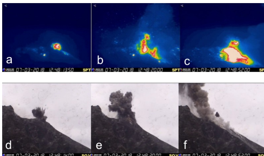
Fig. 3.3 - Immagini significative della sequenza esplosiva del 7 marzo riprese dalla telecamera termica del Pizzo e dalla telecamere visibile di quota 400.
