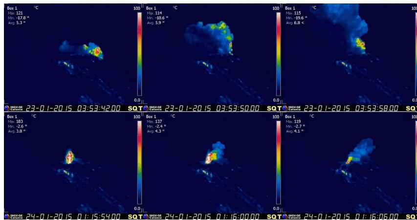
Fig. 1.1 Alcuni fotogrammi dell'esplosione stromboliana più intensa registrata nelle prime ore del 23 gennaio 2015 da una bocca localizzata nell'area craterica meridionale (in alto) e di un'esplosione prodotta dalla bocca localizzata nell'area craterica settentrionale (in basso), registrata nel pomeriggio del 24 gennaio 2015.
