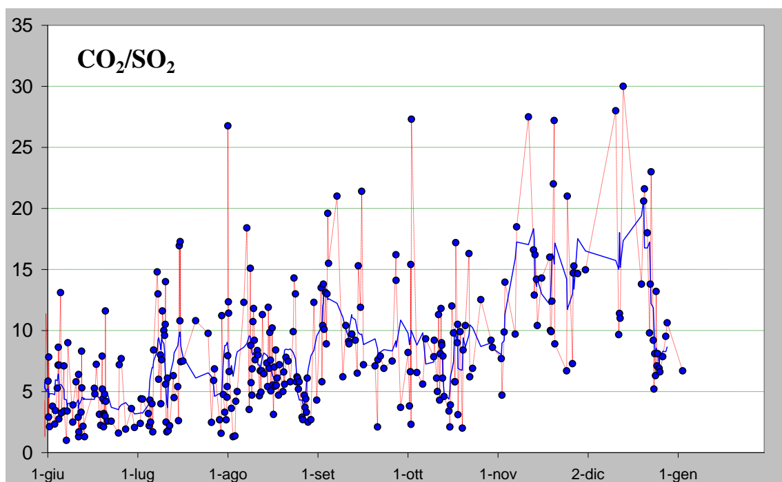
Figura 2– Rapporto \text{CO}_2/\text{SO}_2 misurato nel plume vulcanico dello Stromboli nel periodo tra il 1 giugno e il 3 gennaio 2015 (ultimo dato ore 6:30 locali del 3 gennaio).
