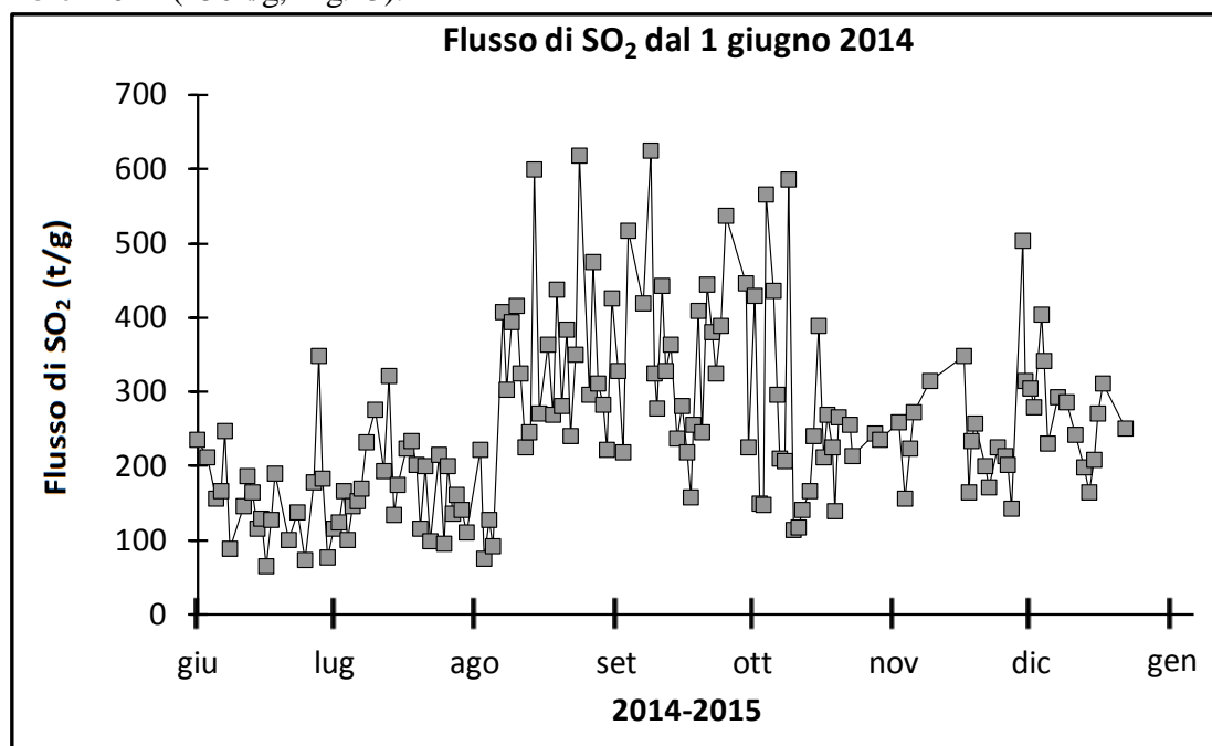
Figura 3 – Flusso di SO 2 medio-giornaliero dal 1 giugno 2014.
