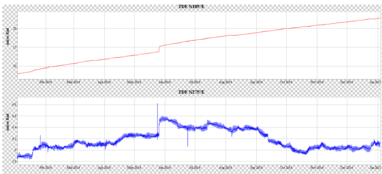
Fig.8- Dato clinometrico nel periodo compreso tra gennaio 2014 e gennaio 2015
