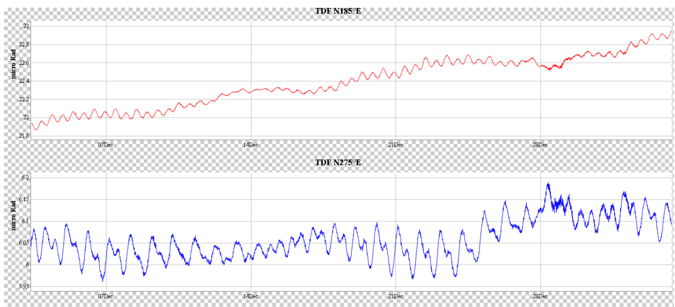
Fig.9 – Dato clinometrico nel periodo compreso tra il 30 novembre 2014 e il 03 gennaio 2015
