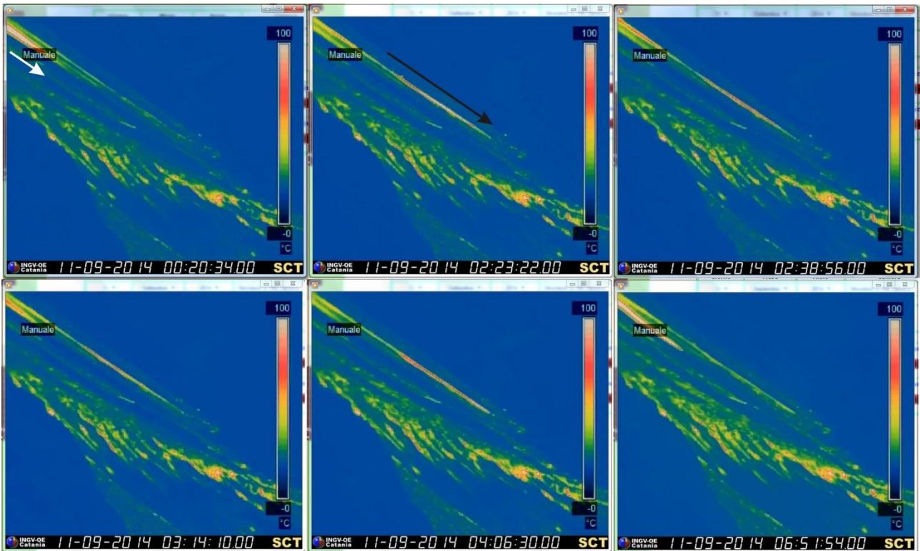
Figura 2 Nelle immagini termiche della telecamera di quota 190 m è visibile l'avanzamento dei fronti lavici: quello descritto nei precedenti comunicati (freccia bianca) e quello formatesi alle ore 02:00 UTC di oggi (freccia nera).
