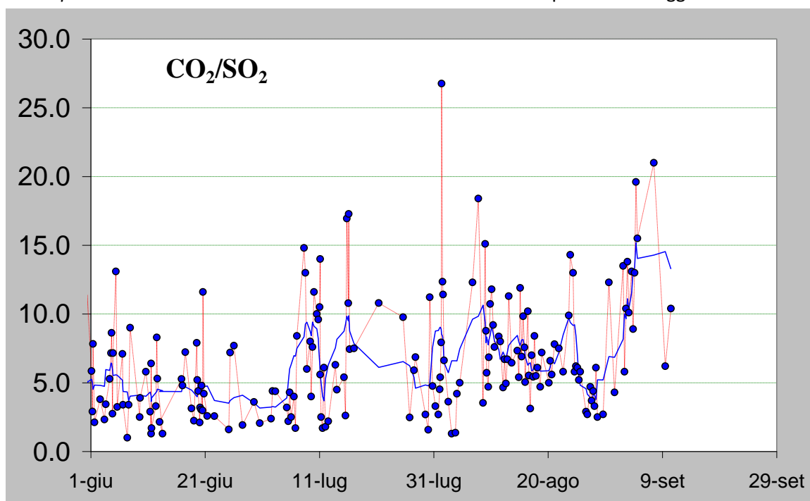
Figura 4 – Rapporto CO 2 /SO 2 misurato nel plume vulcanico dello Stromboli nel periodo tra il 1 giugno ed il 10 settembre 2014 (ultimo dato ore 14:30 locali del 10 settembre).
