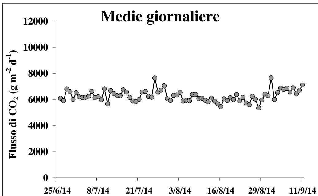
Figura 3 – Flusso medio-giornaliero di CO 2 dal suolo nel periodo tra il 25 giugno ed l'11 settembre 2014
