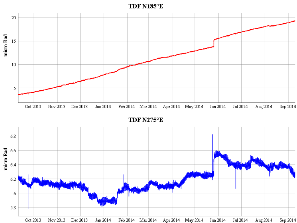
Figura 9 – Dato clinometrico nel periodo compreso tra settembre 2013 e settembre 2014
