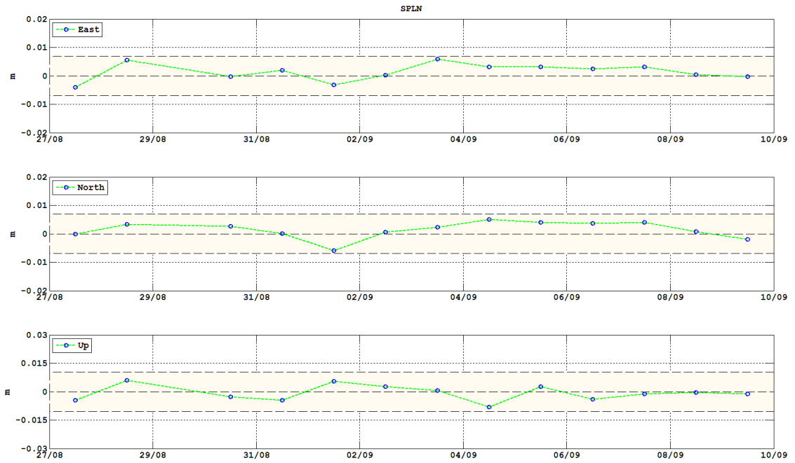
Figura 6 – Dati GPS della stazione di Punta Labronzo del periodo 25/8/2014 – 8/9/2014.
