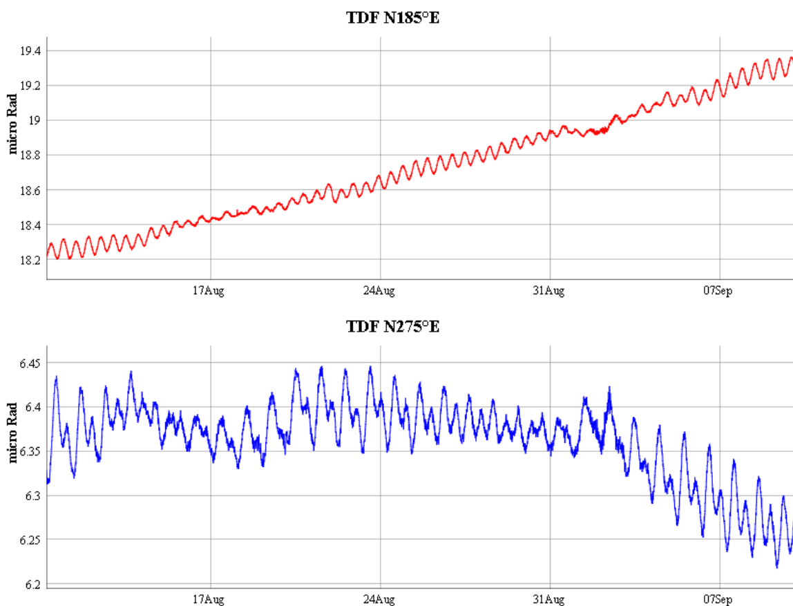
Figura 10 – Dato clinometrico nel periodo compreso tra inizio agosto e il 10 settembre 2014
