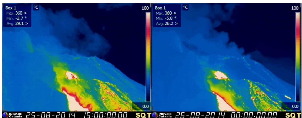
Figura 2 – Immagini termiche della telecamera di quota 400 m s.l.m. acquisite alle ore 15:00 UTC del 25 agosto e alle ore 00:00 UTC di oggi, relative alla parte più elevata del teatro eruttivo. In particolare l'immagine di destra mostra l'aumento dell'area dell'anomalia termica in corrispondenza della bocca eruttiva a partire dalle ore 00:00 UTC di oggi.
