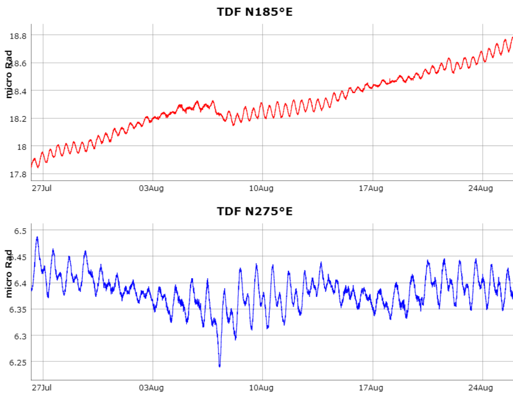
Figura 11 – Dato clinometrico nel periodo compreso tra luglio e il 26 agosto 2014
