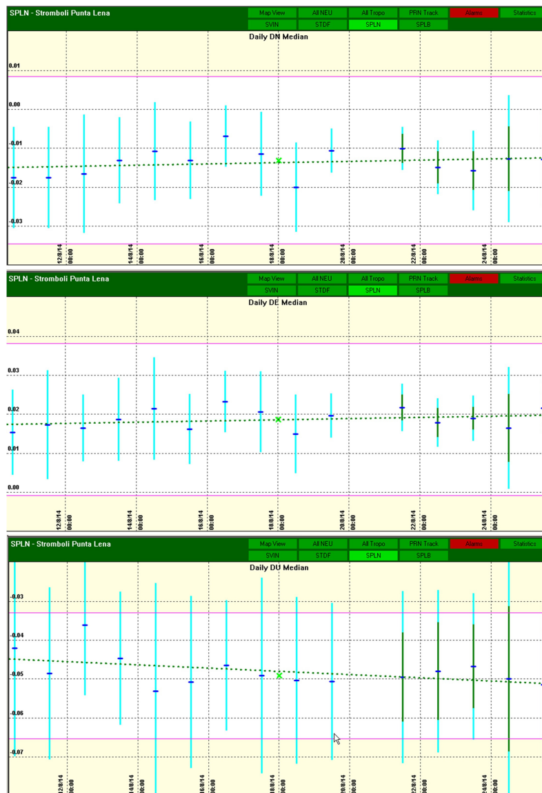
Figura 9 – Dati GPS della stazione di Punta Lena del periodo 3/8/2014 – 25/8/2014.
