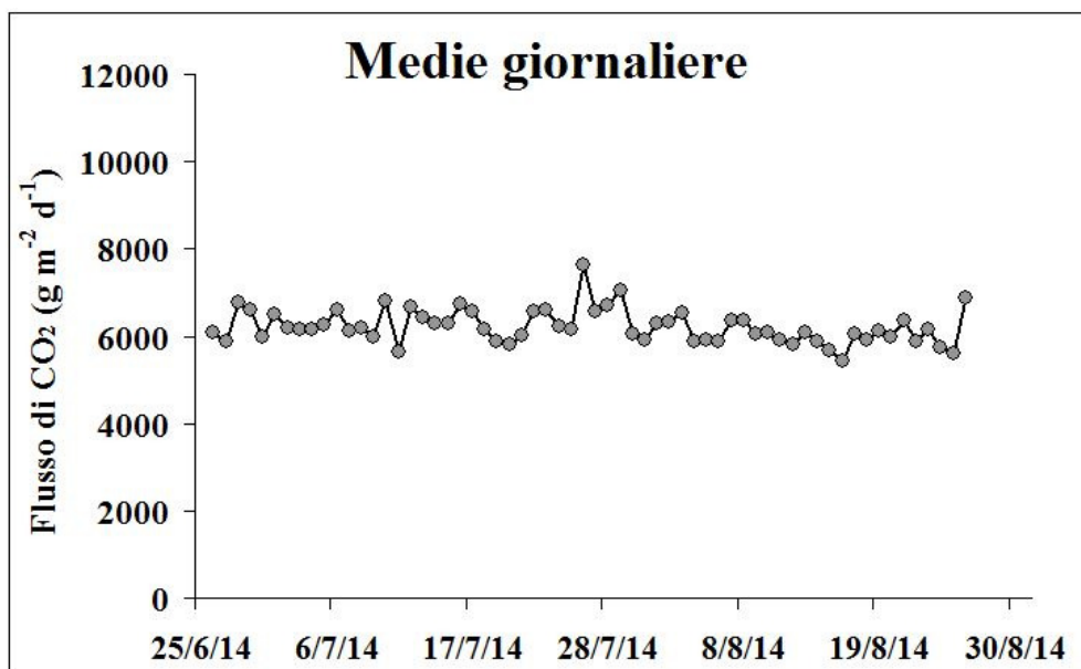
Figura 4 – Flusso medio-giornaliero di CO 2 dal suolo nel periodo tra il 25 giugno ed il 25 agosto 2014
