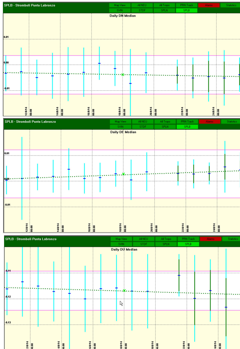
Figura 7 – Dati GPS della stazione di Punta Labronzo del periodo 3/8/2014 – 25/8/2014.
