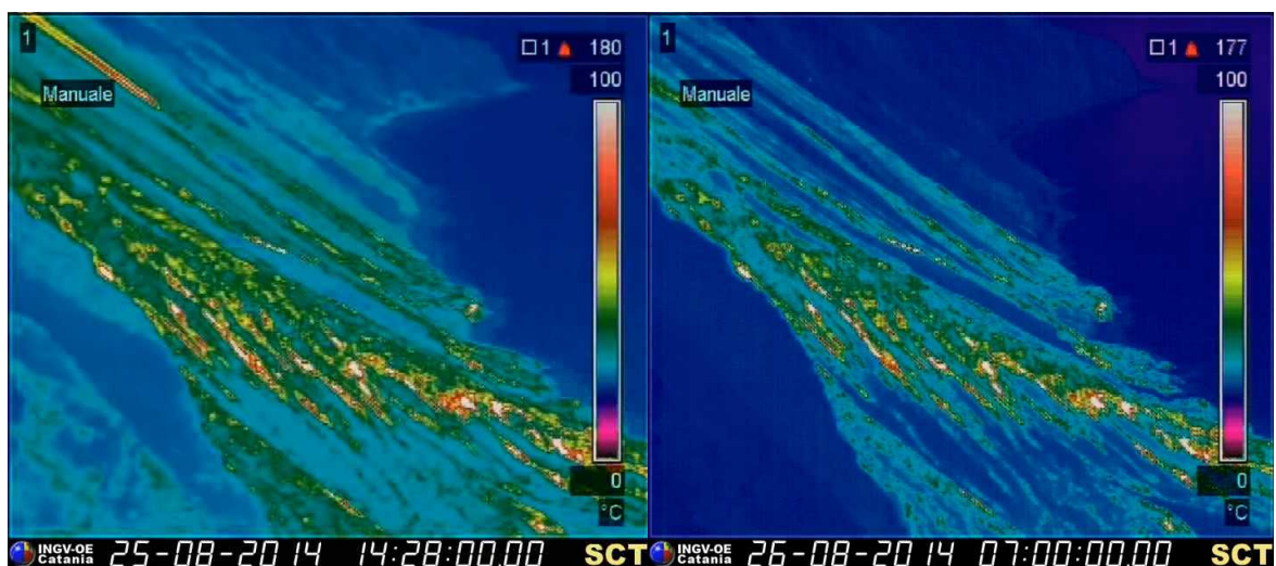
Figura 3 – Immagini termiche della telecamera di quota 190 m s.l.m. Nell'immagine a sinistra si osserva la presenza del fronte lavico che si sviluppa nella parte centrale della Sciara del Fuoco alle ore 14:30 UTC del 25 agosto. L'immagine a destra mostra il campo lavico in raffreddamento ripreso alle ore 07:00 UTC di oggi.
