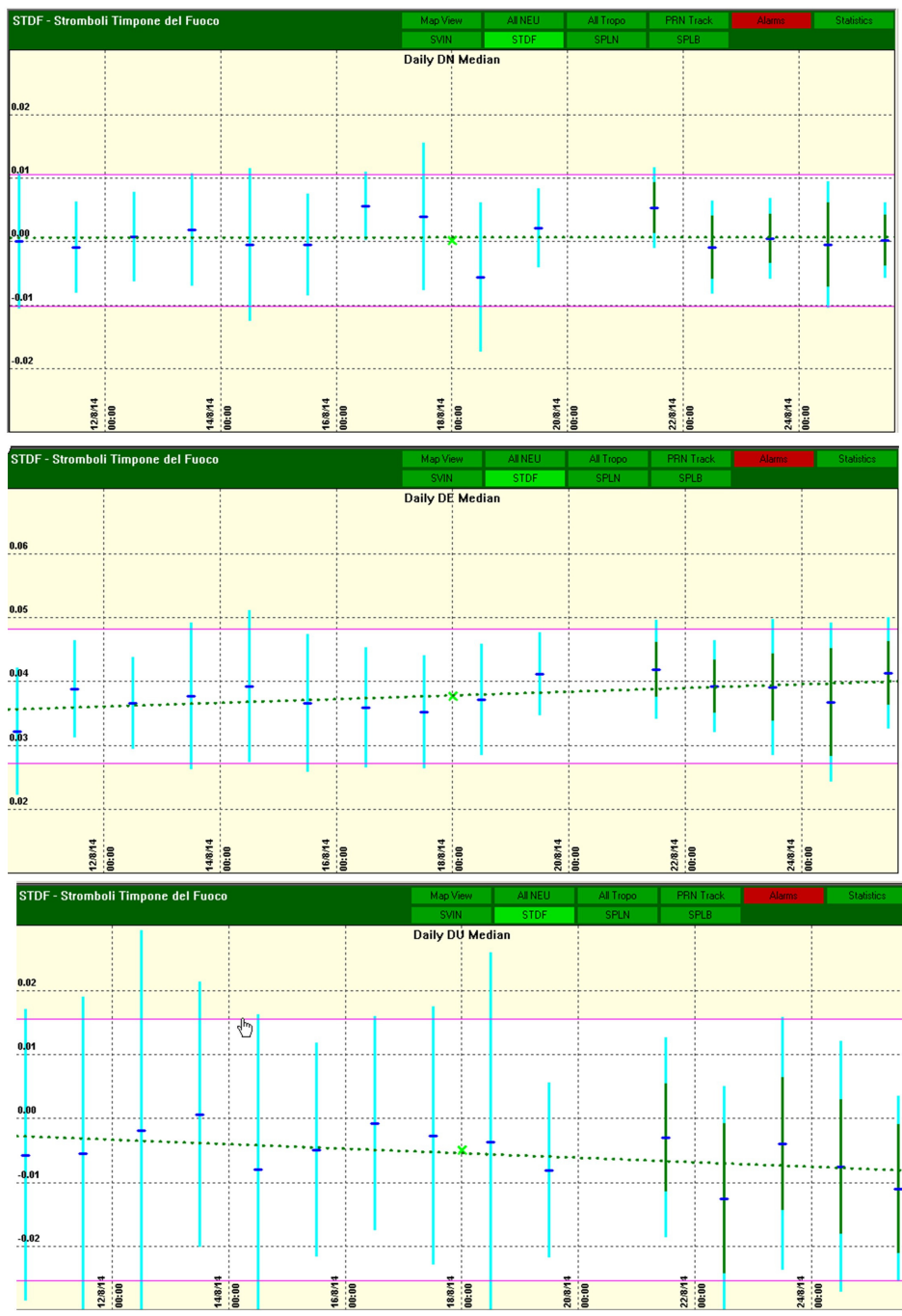
Figura 8 – Dati CGPS della stazione di Timpone del Fuoco del periodo 3/8/2014 – 25/8/2014.
