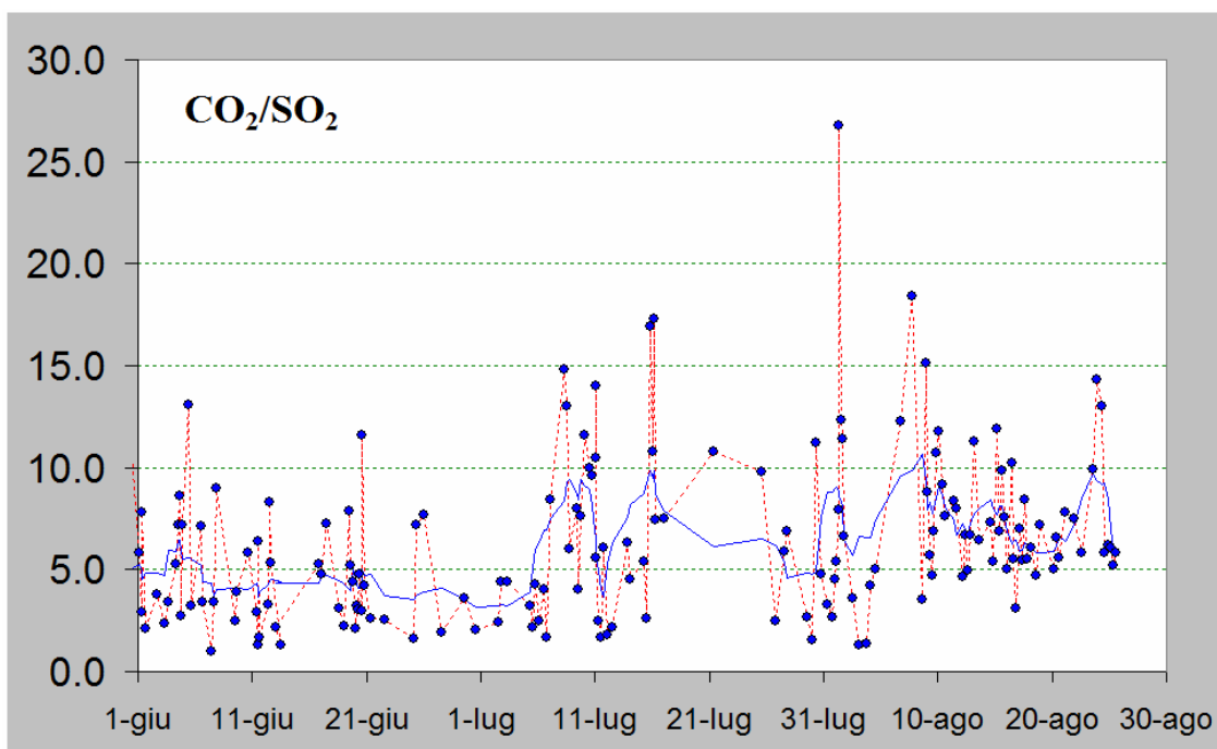
Figura 5– Rapporto CO 2 /SO 2 misurato nel plume vulcanico dello Stromboli nel periodo tra il 1 giugno ed il 25 agosto 2014 (ultimo dato ore 15:30 locali del 25 agosto).
