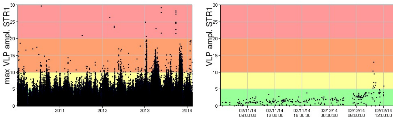
Fig. 4.4 Ampiezza dei VLP alla stazione STR1 dal 1/1/2010 (sinistra) ed ampiezza dei VLP alla stazione STR1 relativa ai soli due giorni (11-12/02) a causa di problemi tecnici al sistema di elaborazione dei dati.
