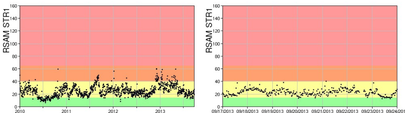
Fig. 4.2 Media giornaliera dell'ampiezza del tremore alla stazione STR1 dal 1/01/2010 (sinistra)
