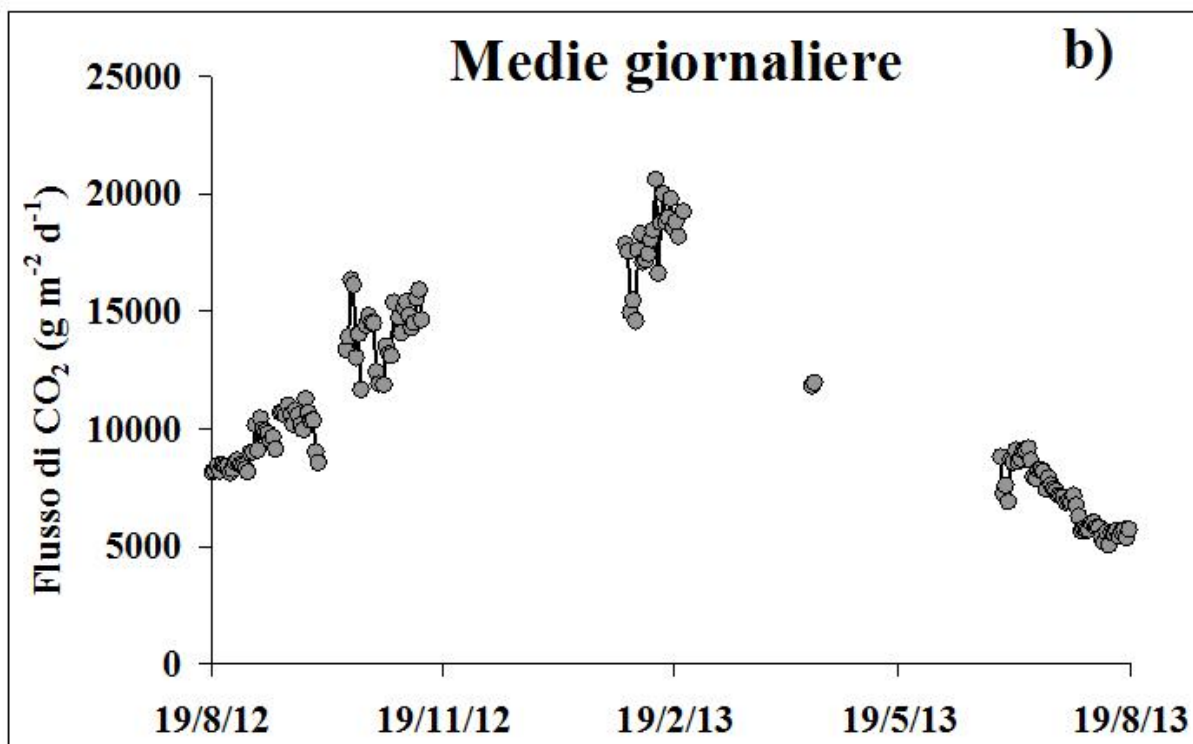
Fig. 2.1 Andamento temporale del flusso di CO 2 dai suoli: a) ultimi due mesi; b) ultimo anno
