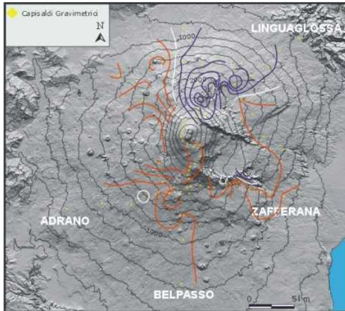
Fig. 2 - Rappresentazione areale delle variazioni gravimetriche osservate nel periodo giugno 2007 – luglio 2008 nella rete dell'Etna (equidistanza = 10 \mu\text{Gal} ). Gli errori sulle variazioni gravimetriche sono compresi entro \pm 10 \mu\text{Gal} ; errori più consistenti interessano le variazioni gravimetriche lungo il Profilo Sommitale (entro \pm 15 \mu\text{Gal} ).
