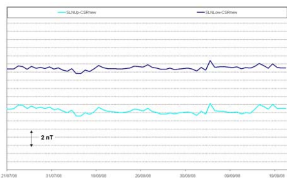
Fig. 12 – Differenze delle medie giornaliere dell'intensità totale registrate alle stazioni di SPL e SPC, riferite a CSR.
