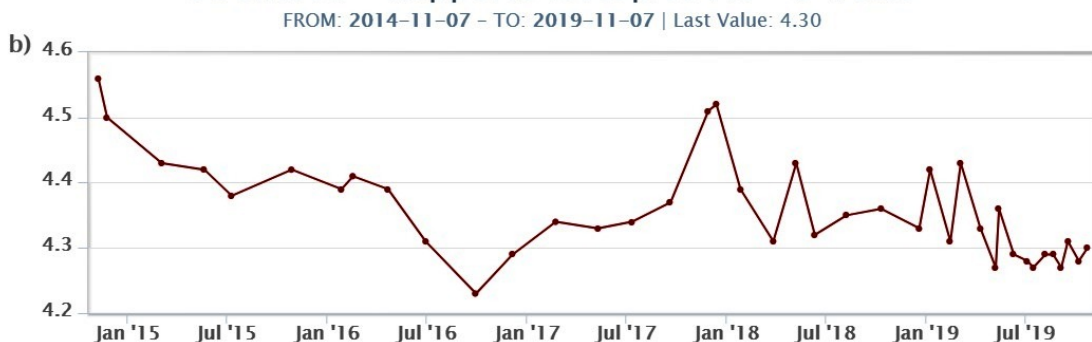
Fig. 6.3 - Andamento temporale medio del rapporto isotopico dell'elio disciolto nella falda termale: a) ultimo anno; b) ultimo quadriennio.
