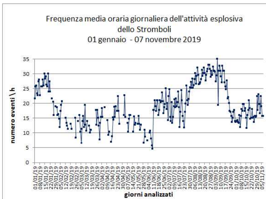
Fig. 3.2 - Frequenza media oraria giornaliera totale delle esplosioni dello Stromboli tra gennaio e 7 novembre 2019
