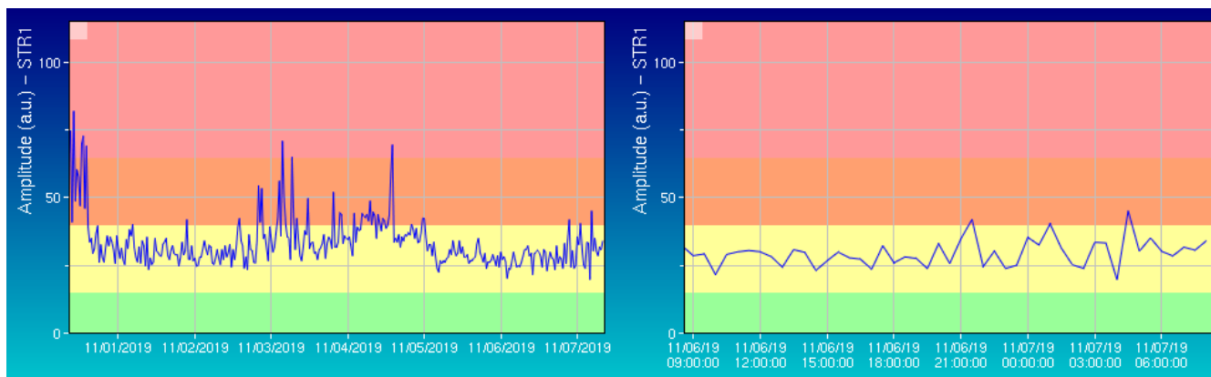
Fig. 4.2 - Ampiezza del tremore alla stazione STR1 nell'ultima settimana (sinistra) e nelle ultime 24 ore (destra).
