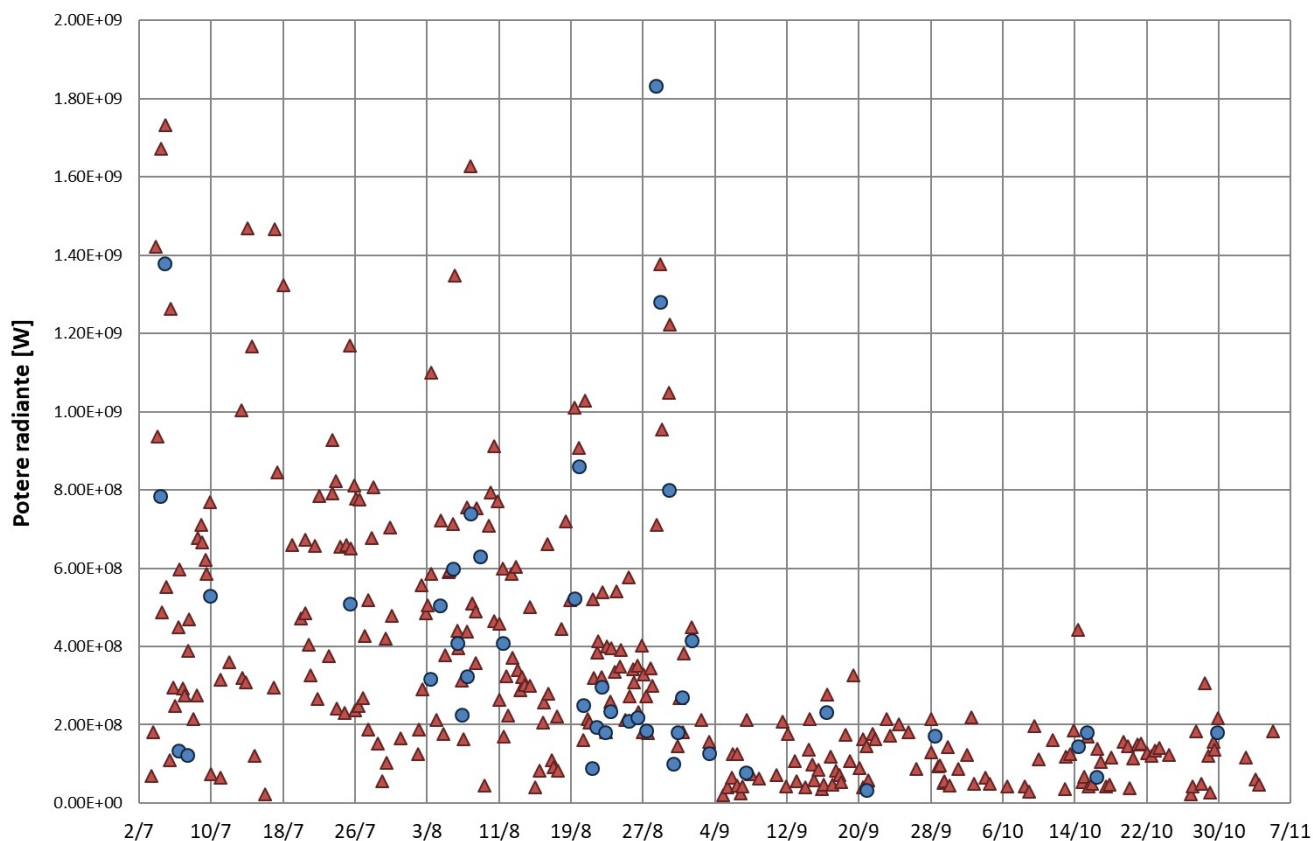
Fig. 7.1 - Flusso radiante calcolato da dati MODIS (triangolo rosso) e Sentinel-3 SLSTR (cerchio blu) dal 3 luglio al 5 novembre.
