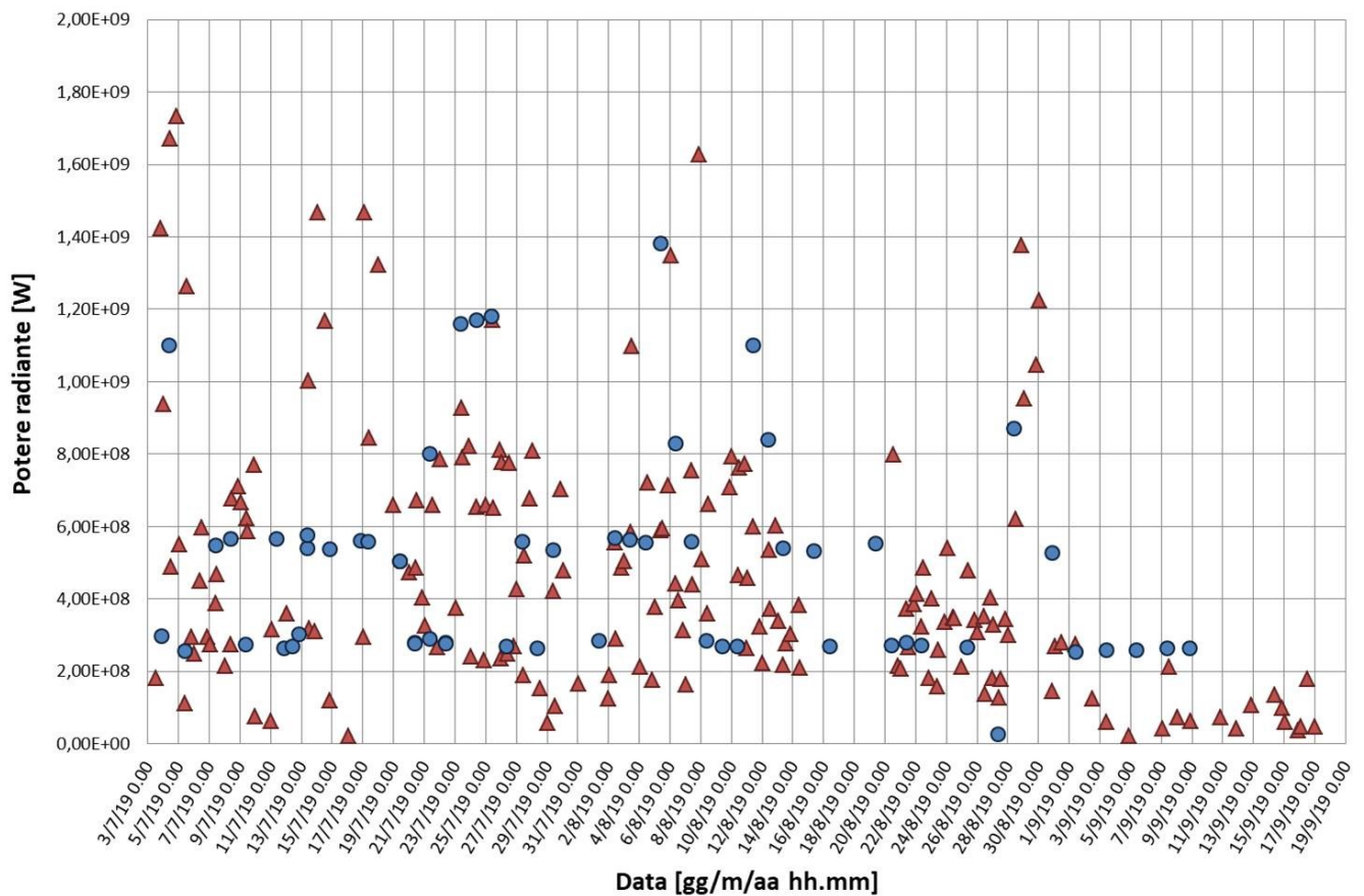
Fig. 7.1 - Flusso radiante calcolato da dati MODIS (triangolo rosso) e Sentinel-3 SLSTR (cerchio blu) dal 3 luglio al 17 settembre.
