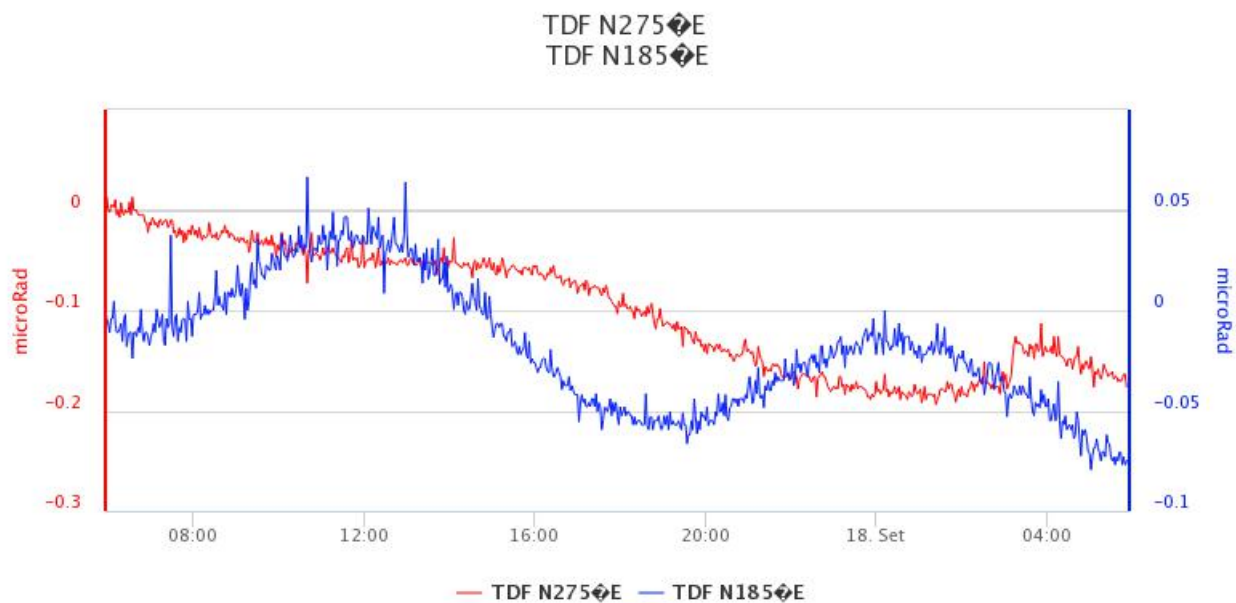
Fig. 5.2 - Serie temporale delle componenti X e Y della stazione TDF
