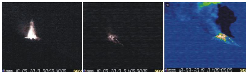
Fig. 3.1 - Immagini dell'attività stromboliana dalle bocche presenti nell'area craterica N (a sinistra) con ricaduta del materiale esplosivo sui fianchi dell'area craterica (al centro), visibile anche dalle immagini della telecamera termica (a destra). Immagini riprese dalle telecamere di quota 400 m, il 18 settembre 2019.
