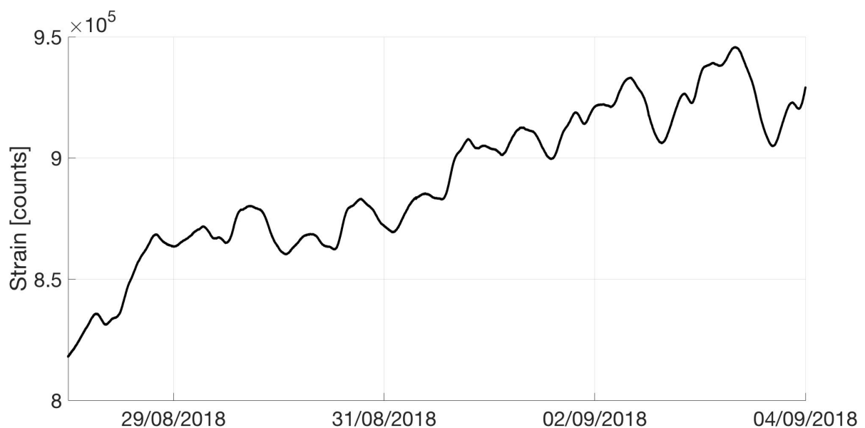
Fig. 4.3 - Grafico relativo ai dati dilatometrici registrati a SVO: in nero viene mostrato il dato processato, ripulito dalle maree.
