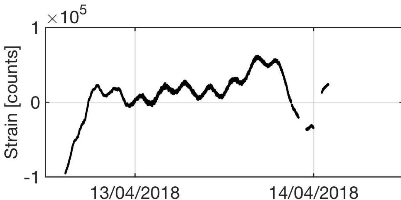
Fig. 4.4 - Grafico relativo ai dati dilato metrici registrati a SVO: viene mostrato il dato processato ripulito dalle maree e dalla pressione atmosferica.
