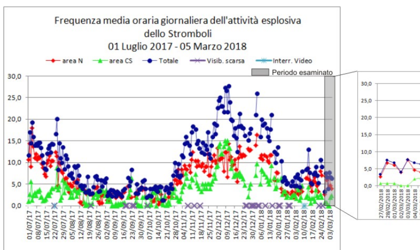
Fig. 3.2 - Nel grafico è visualizzata la frequenza oraria media giornaliera degli eventi esplosivi ripresi dalle telecamere di sorveglianza dal 01 Luglio 2017. La depressione craterica è stata suddivisa in aree sede di bocche eruttive attive (vedi Fig. 3.1). Il valore Totale è la somma della frequenza oraria media
