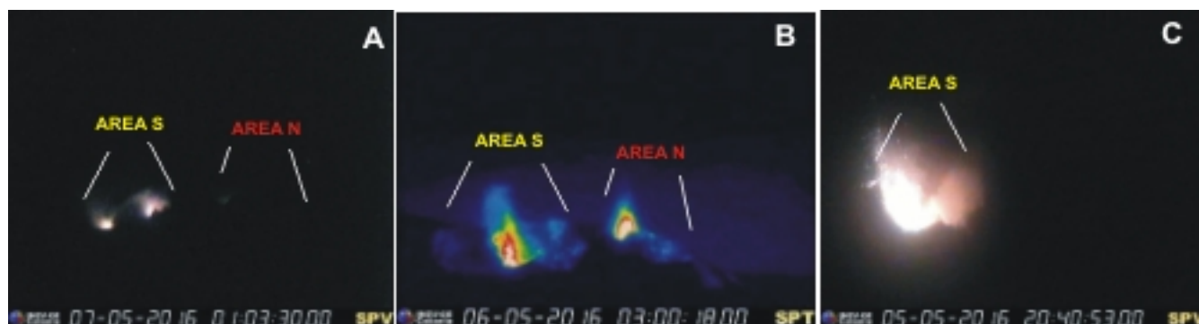
Fig. 1.1 La terrazza craterica ripresa dalla telecamera in banda visibile (A e C) e termica (B) del Pizzo sopra la Fossa. In A) si osservano le due bocche attive nell'area craterica meridionale e in B) si vede anche un'esplosione dalla bocca attiva nell'area craterica settentrionale. In C) si osserva un'esplosione con lancio di brandelli di lava da una delle due bocche presenti nell'area craterica meridionale.
