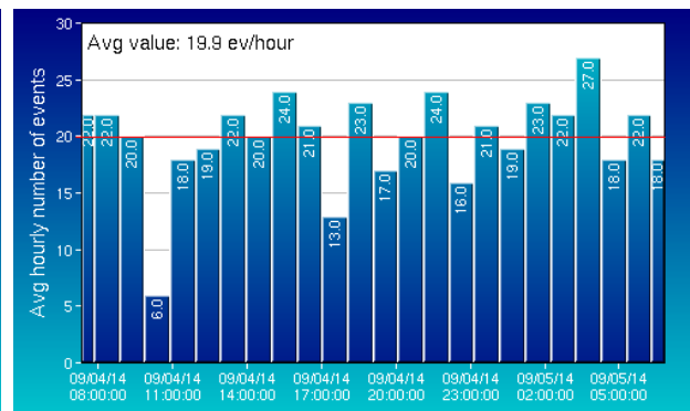
Frequenza giornaliera di accadimento degli eventi VLP nell'ultima settimana (sinistra) e nelle ultime 24h
