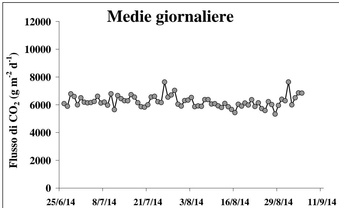
Figura 4 – Flusso medio-giornaliero di \text{CO}_2 dal suolo nel periodo tra il 25 giugno ed il 5 settembre 2014
