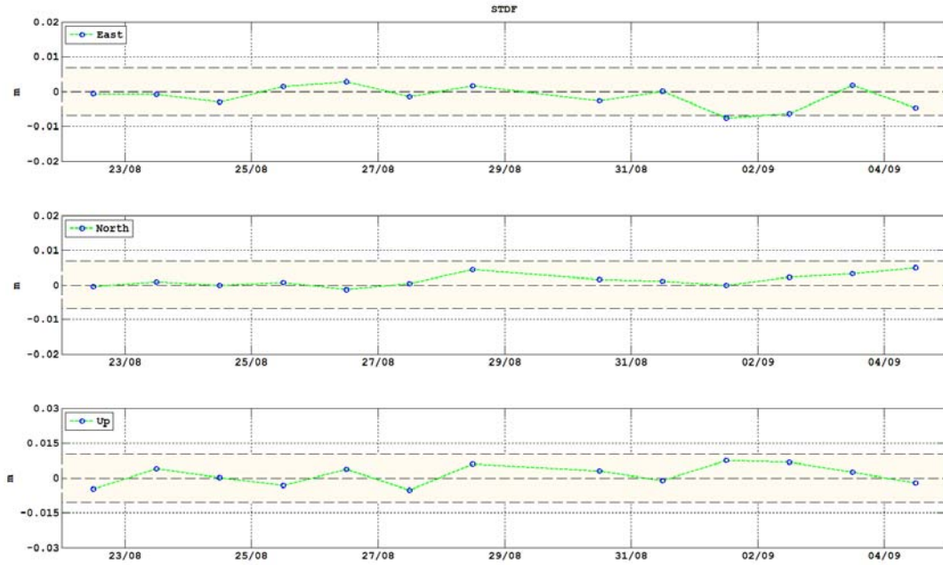
Figura 8 – Dati CGPS della stazione di Timpone del Fuoco del periodo 18/8/2014 – 5/9/2014.
