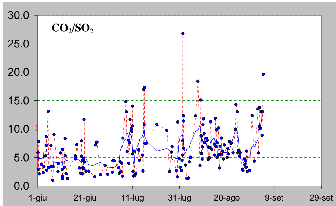
Figura 5 – Rapporto \text{CO}_2/\text{SO}_2 misurato nel plume vulcanico dello Stromboli nel periodo tra il 1 giugno ed il 4 settembre 2014 (ultimo dato ore 11:30 locali del 4 settembre).
