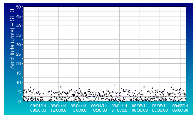
Ampiezza dei VLP alla stazione STR1 nell'ultima settimana (sinistra) e nelle ultime 24h
