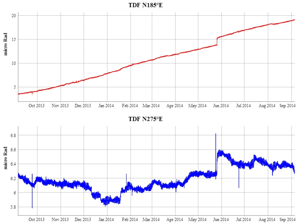
Figura 10 – Dato clinometrico nel periodo compreso tra agosto 2013 e settembre 2014
