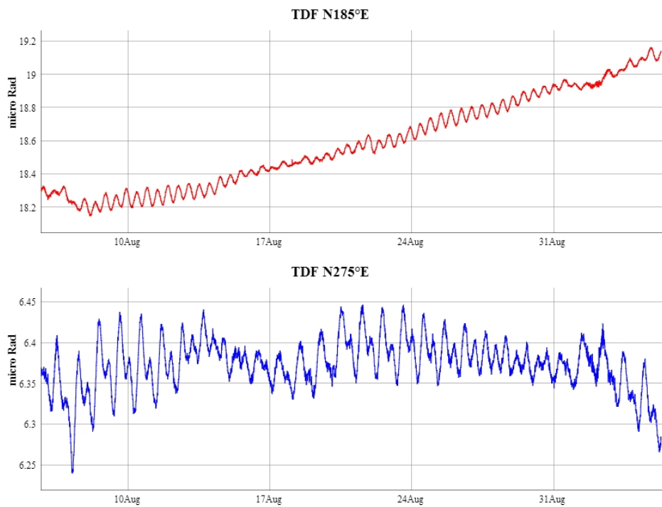
Figura 11 – Dato clinometrico nel periodo compreso tra inizio agosto e il 5 settembre 2014
