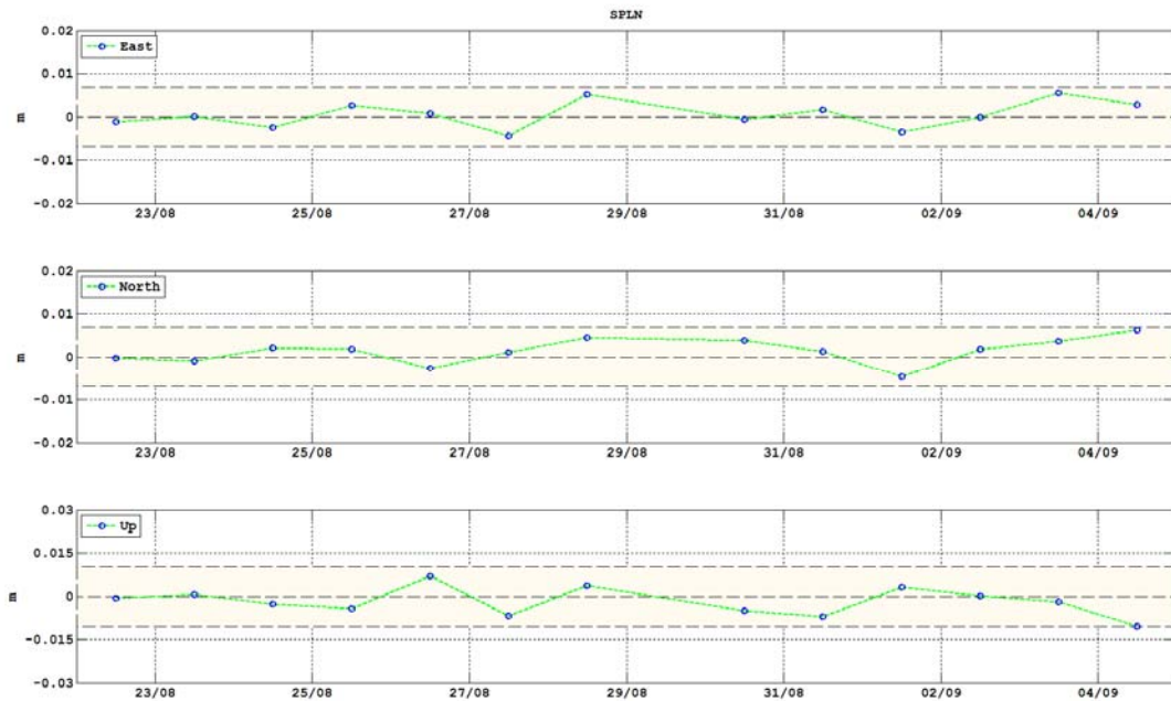
Figura 9 – Dati GPS della stazione di Punta Lena del periodo 18/8/2014 – 5/9/2014.
