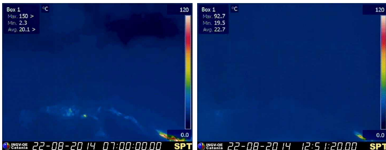
Figura 1 – Immagini termiche della telecamera del Pizzo, acquisite questa mattina e nel primo pomeriggio, relative all'area craterica sommitale. Nonostante la visibilità sia rimasta parziale per alcuni tratti della mattinata, si apprezza la sostanziale costanza del quadro eruttivo, con un'area termicamente rilevante in corrispondenza della bocca effusiva (nelle immagini in basso a destra).
