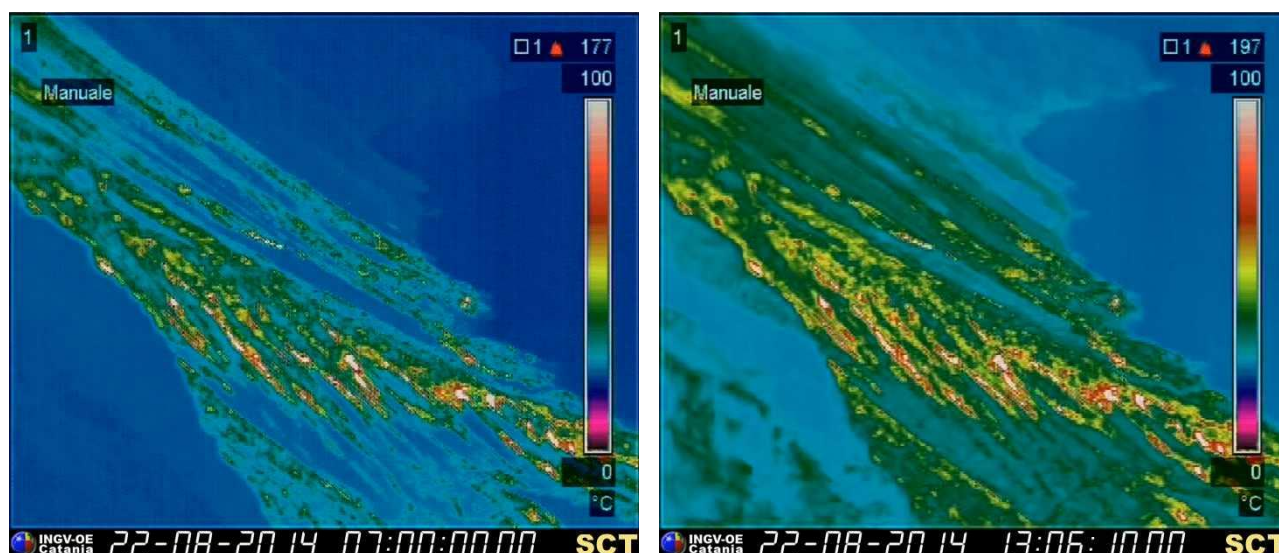
Figura 3 – Immagini termiche dalla telecamera di quota 190 m s.l.m. che mostrano il campo lavico in raffreddamento nella zona più bassa della Sciara del Fuoco.
