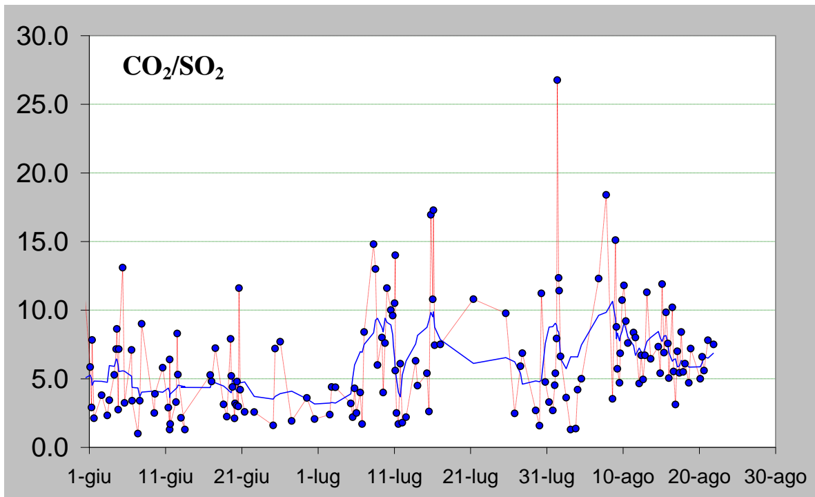
Figura 5– Rapporto CO 2 /SO 2 misurato nel plume vulcanico dello Stromboli nel periodo tra il 1 giugno ed il 21 agosto 2014 (aggiornato alle ore 23:30 locali)
