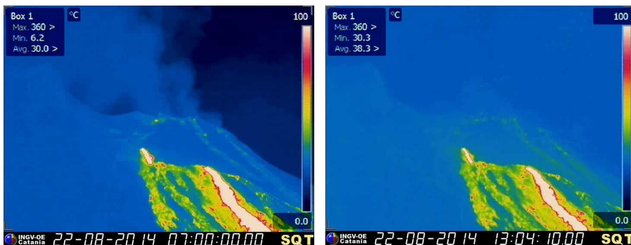
Figura 2 – Immagini termiche della telecamera di quota 400 m s.l.m. acquisite questa mattina e nel primo pomeriggio, relative alla parte più elevata del teatro eruttivo. Tali immagini mostrano la persistenza del trabocco lavico centrale lungo la Sciara del Fuoco.
