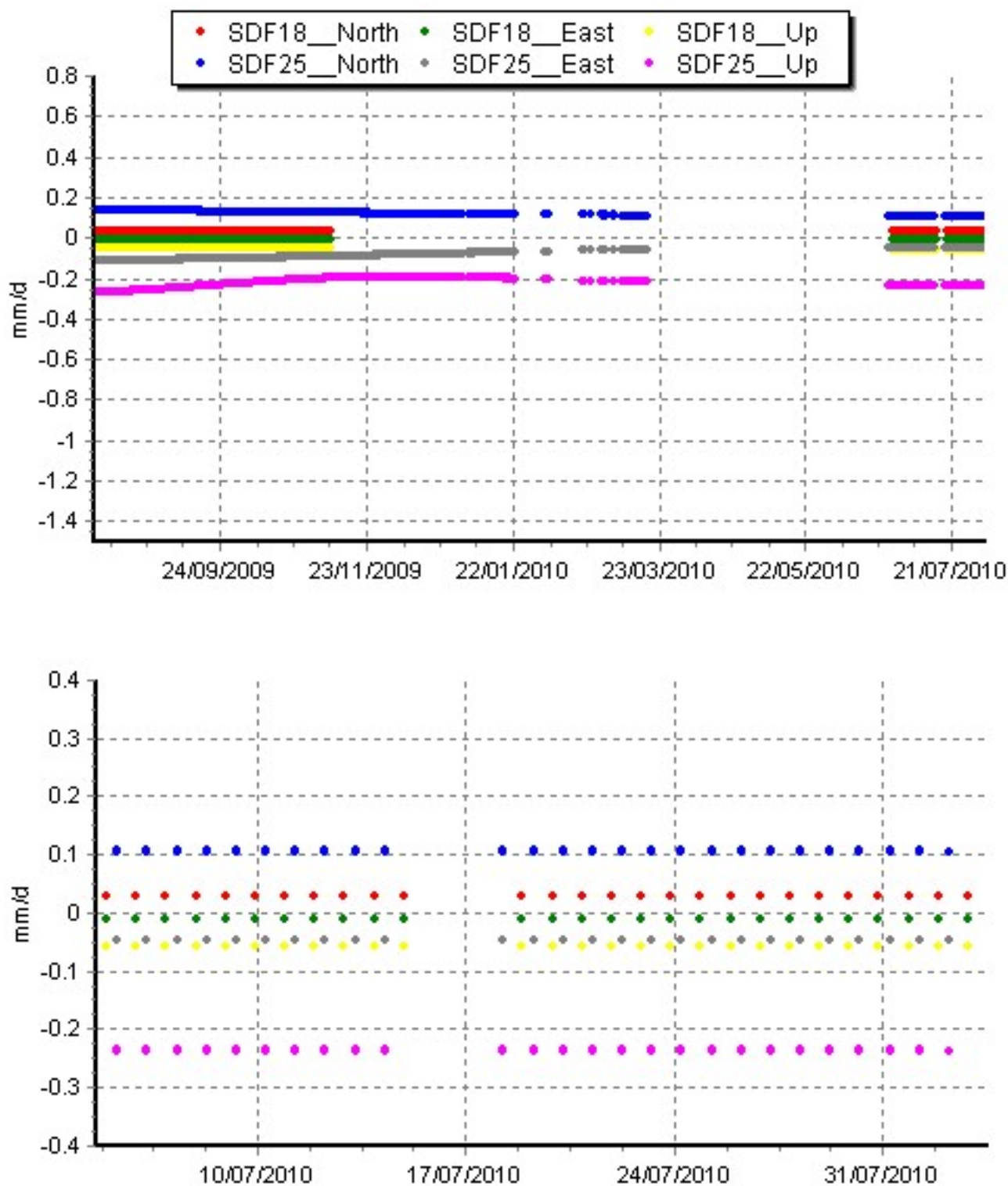
Fig. 3.2 Variazione delle Velocità di Deformazione verticale e orizzontale (nelle due componenti Nord e Est) di due capisaldi del sistema THEODOROS (SDF18 e SDF25). Le velocità, medie giornaliere, sono misurate in mm/giorno. I periodi considerati nei grafici sono di un anno (in alto) ed un mese (in basso).
