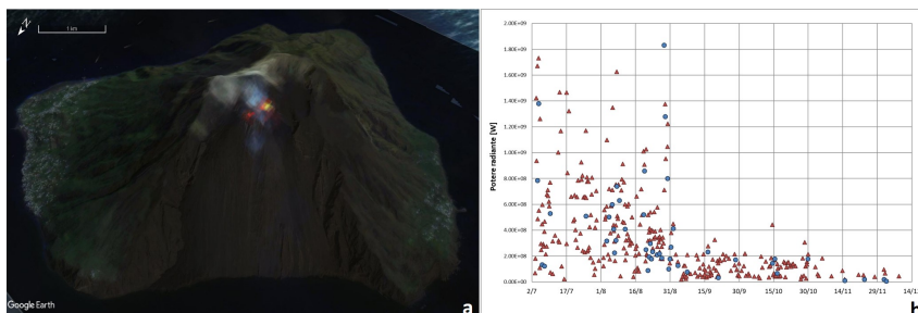
Fig. 7.1 - a) RGB composita delle bande 12, 11 e 5 dell'immagine Sentinel-2 del 4 dicembre 2019, 09h:54m GMT (risoluzione spaziale 20m), in cui è visibile l'anomalia termica associata all'attività sommitale. b) Flusso radiante calcolato da dati MODIS (triangolo rosso) e Sentinel-3 SLSTR (cerchio blu) dal 3 luglio al 8 dicembre.
