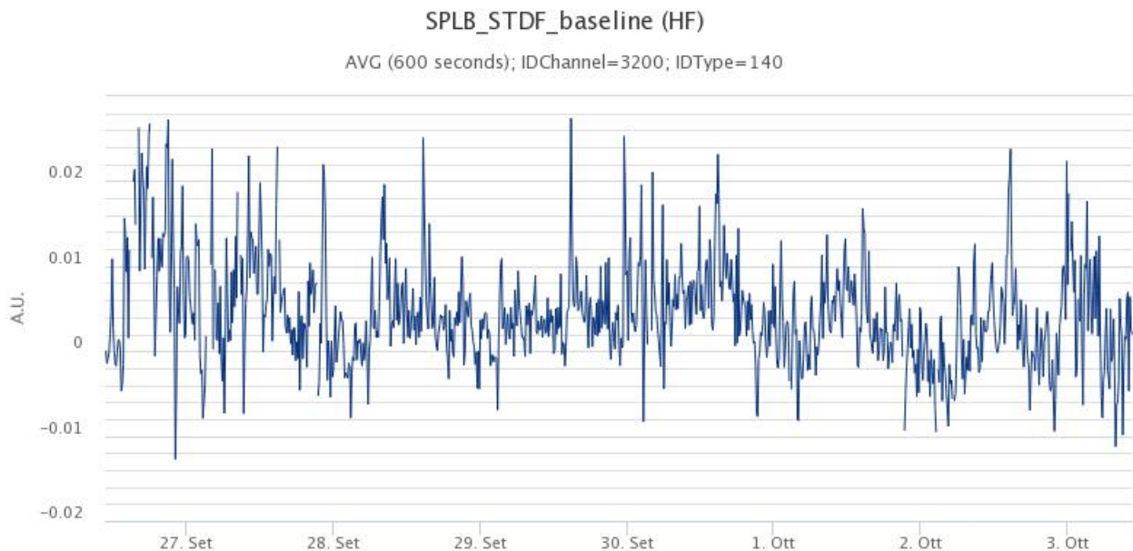
Fig. 5.1 - Serie temporale della variazione della distanza STDF-SPLB
