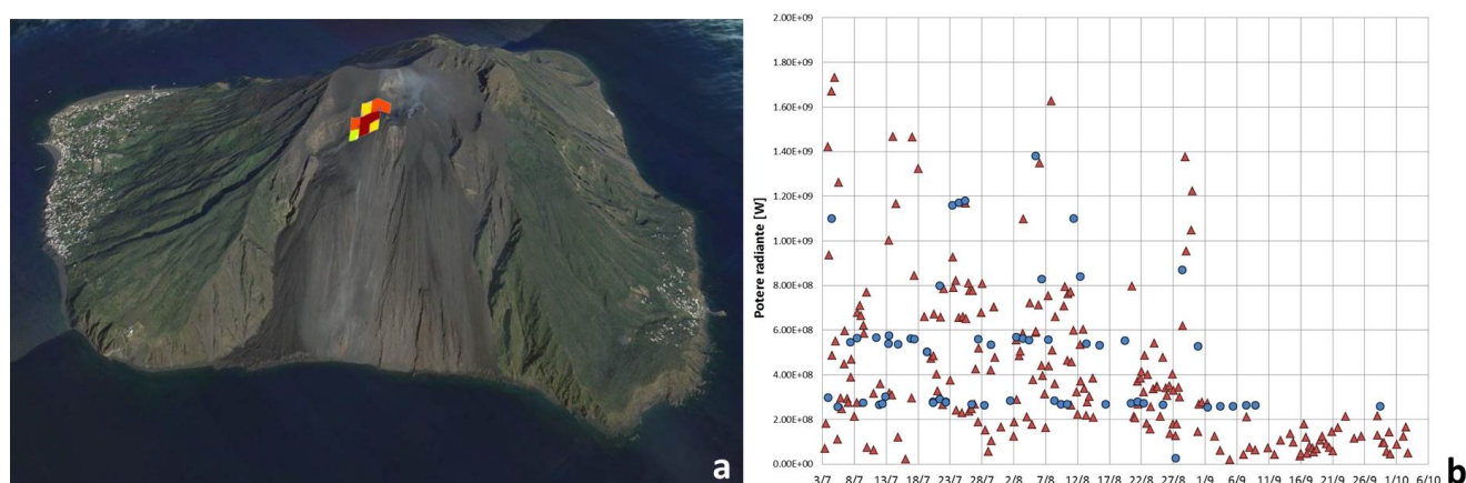
Fig. 7.1 - Fig. 7.1 –a) Mappa delle anomalie termiche ricavate dall'immagine ECOSTRESS del 1 ottobre alle 13h46m GMT b) Flusso radiante calcolato da dati MODIS (triangolo rosso) e Sentinel-3 SLSTR (cerchio blu) dal 3 luglio al 2 ottobre
