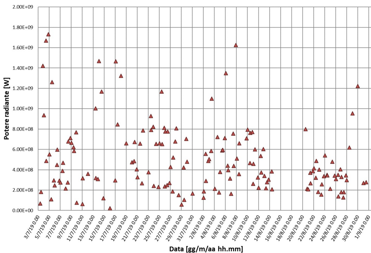
Fig. 7.1 - Flusso radiante a Stromboli calcolato da dati MODIS dal 3 luglio al 31 agosto 2019
