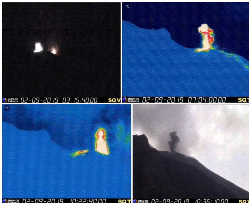
Fig. 3.1 - Fig. 3.1. Immagini sul visibile e sul termico registrate dalle telecamere di quota 400 nella mattinata del 2 settembre 2019, che mostrano in maniera rappresentativa l'attività esplosiva osservata durante le ultime 24 ore.
